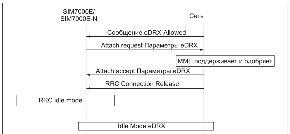
Рис. 5. Процедура перехода в режим eDRX
