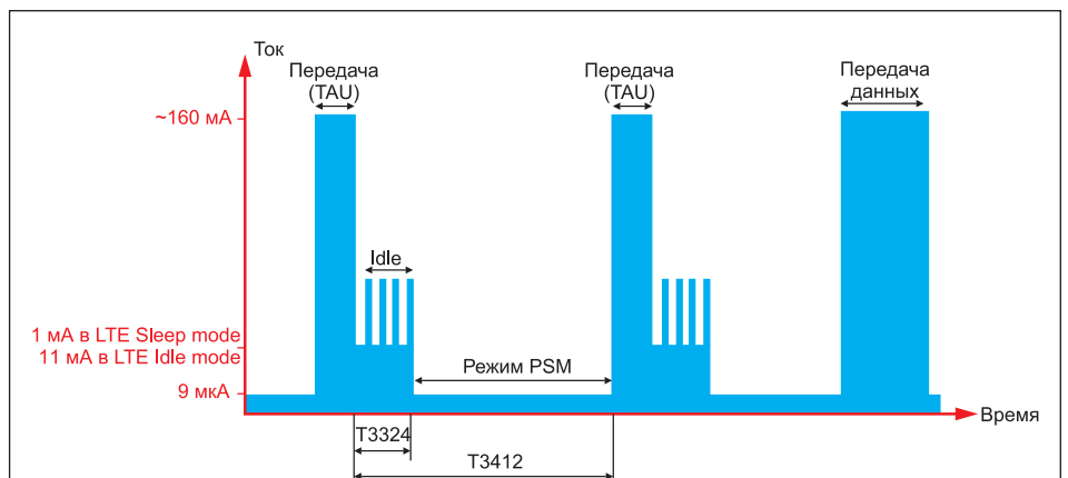
Рис. 6. Потребление тока модулем в режиме PSM
