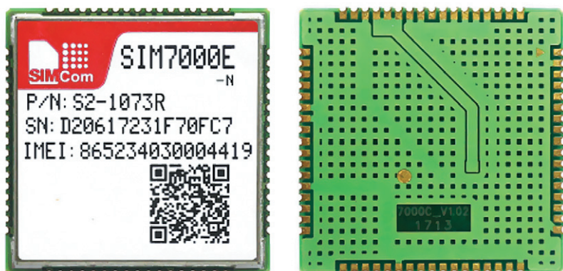
Рис. 3. Мультидиапазонный NB-IoT/GSM-модуль SIM7000E-N (слева — вид сверху, справа — вид снизу)
