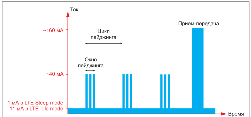
Рис. 4. Потребление тока модулем в режимах LTE Sleep/LTE Idle и во время обмена данными с сетью
