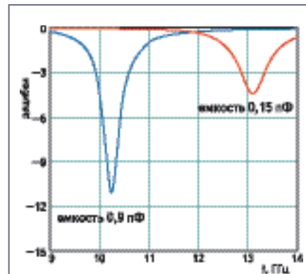
Рис. 4. Амплитуда коэффициента отражения ячейки микрополоскового элемента; расчеты выполнены по эквивалентной схеме в программе Ansoft Designer
