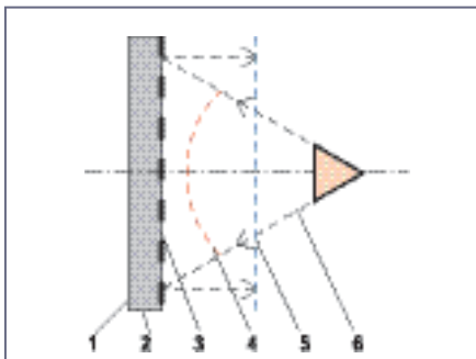
Рис. 1. Микрополосковая отражательная антенная решетка: 1 — металлический экран; 2 — диэлектрическая плата; 3 — элемент «излучатель – фазовращатель»; 4 — сферический фронт падающей волны из облучателя; 5 — плоский фронт, сформированный антенной; 6 — облучатель
