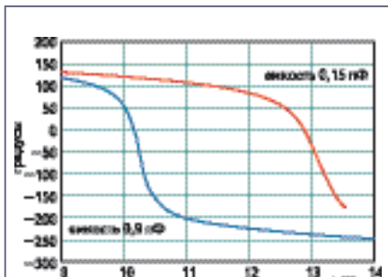
Рис. 3. Фаза коэффициента отражения ячейки микрополоскового элемента с включенным в него варактором; расчетная кривая выполнена по программе Ansoft Designer
