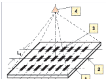
Рис. 2. Общий вид отражательной антенной решетки с электрическим сканированием: 1 — диэлектрик; 2 — экран; 3 — элемент «излучатель – фазовращатель»; 4 — облучатель
