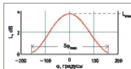
Рис. 5. Экспериментальные данные потерь в зависимости от фазового угла на частоте 12 ГГц; варактор MA46H120 с добротностью Q=3000
