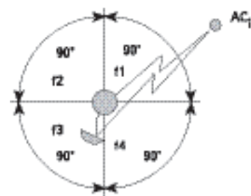
Рис. 3. Влияние отражающих поверхностей: f_1 = f_3 — пример неверного частотного планирования; f_1 \neq f_3 — пример правильного частотного планирования
