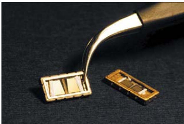
Рис. 5. Фото квазиеверных фильтров на ПАВ на базе ОНВШП фильтров в металлокерамическом SMD-корпусе 13,3×6,5 мм (не закрытые)
