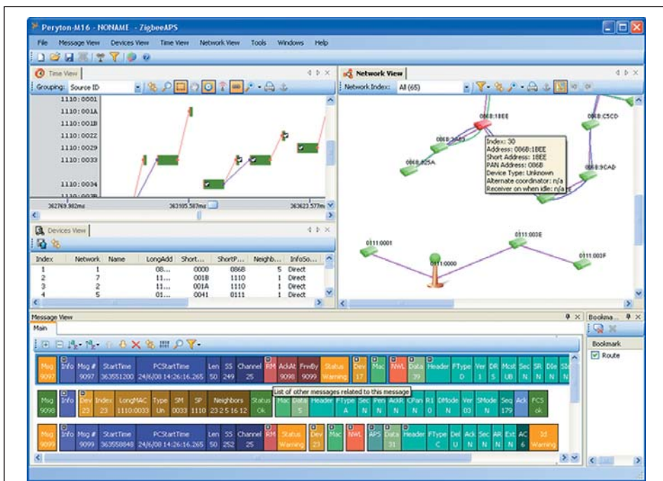
Рис. 3. Анализатор трафика сетей ZigBee от компании Perytons
