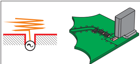
Рис. 2. Спиральный монополь
