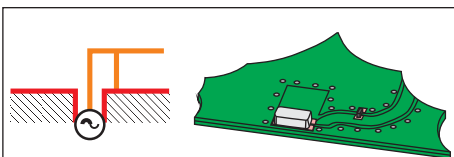
Рис. 3. Керамическая PIFA-антенна
