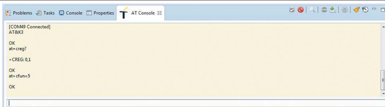
Рис. 7. Консоль AT-команд
