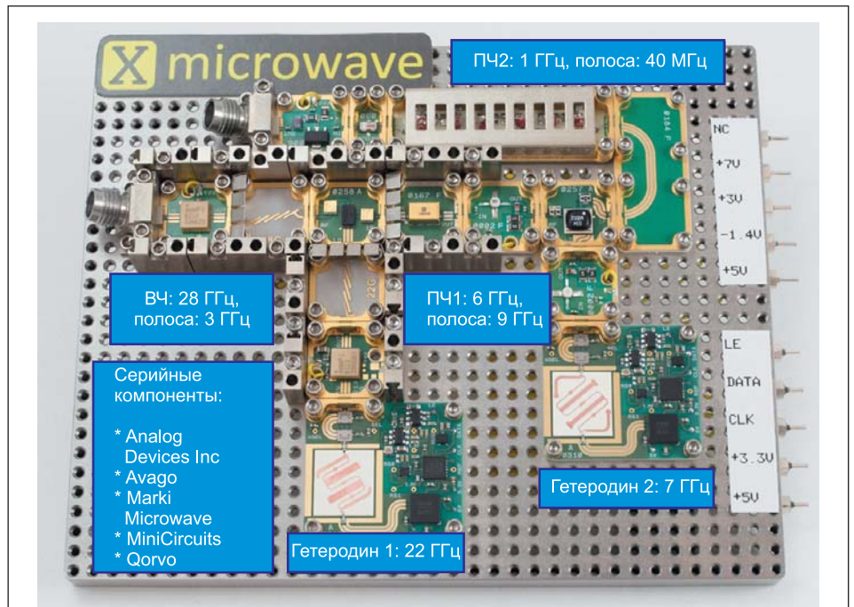
Рис. 3. Аппаратный прототип приемника 28 ГГц, использующий X-блоки из X-Microwave
