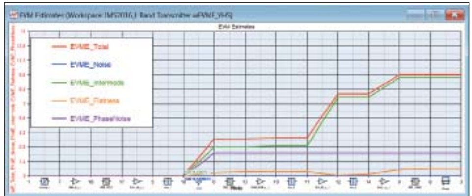
Рис. 2. Новейший метод анализа амплитуды вектора ошибки позволяет выявить компоненты, вызывающие деградацию ВЧ-сигналов с цифровой модуляцией, и исключить дорогостоящие итерации в процессе создания прототипа
