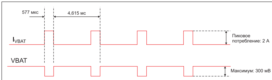
Рис. 6. Потребление модулей SIM7600 и максимально допустимые просадки на шине питания
